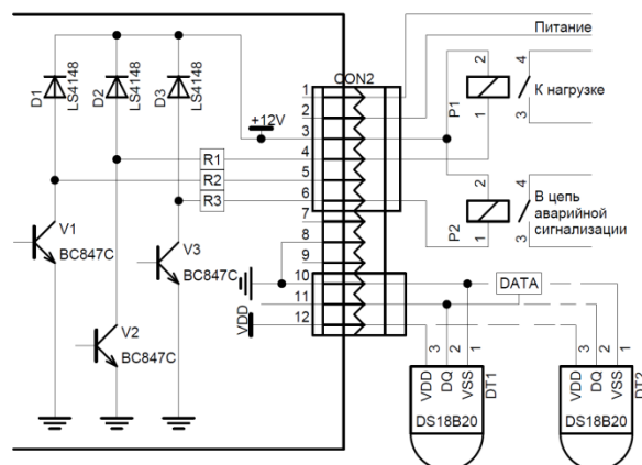
Подключение нескольких датчиков только для модели 3010/3020
